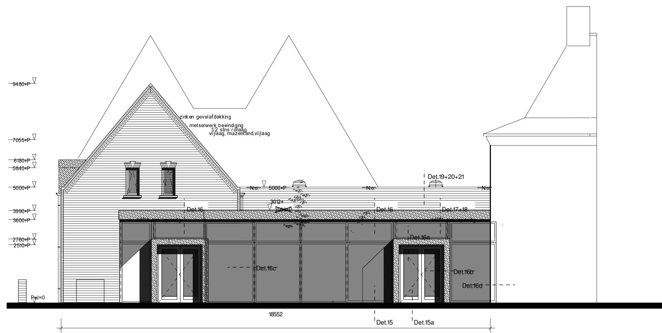
Voorgevel NIEUW
