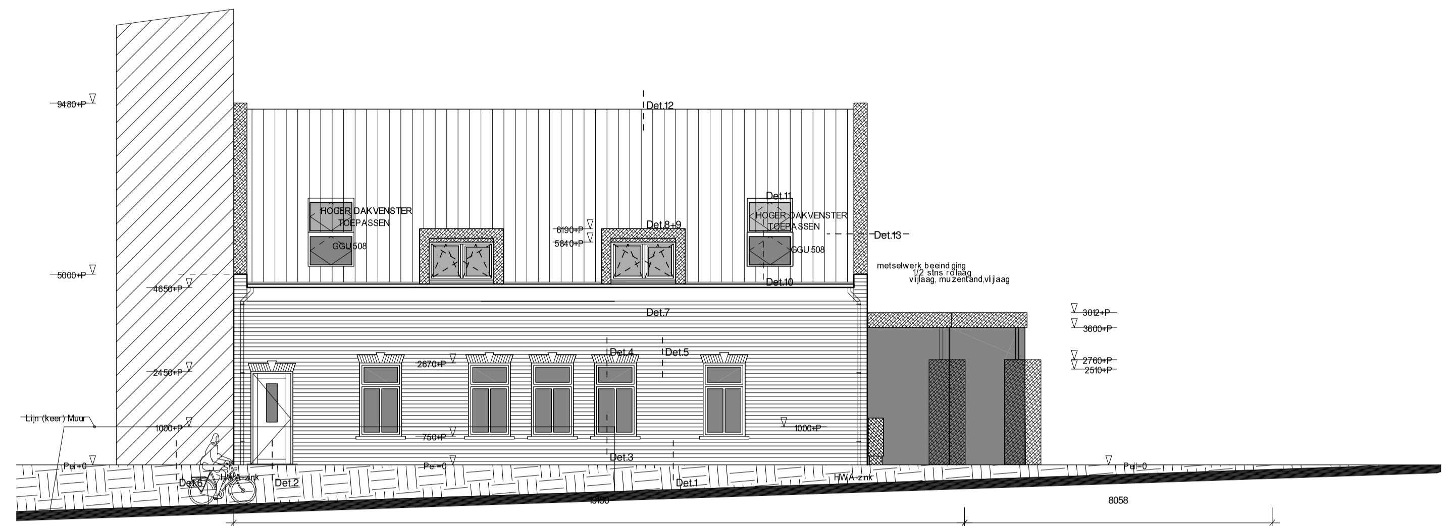
Zijgevel NIEUW
