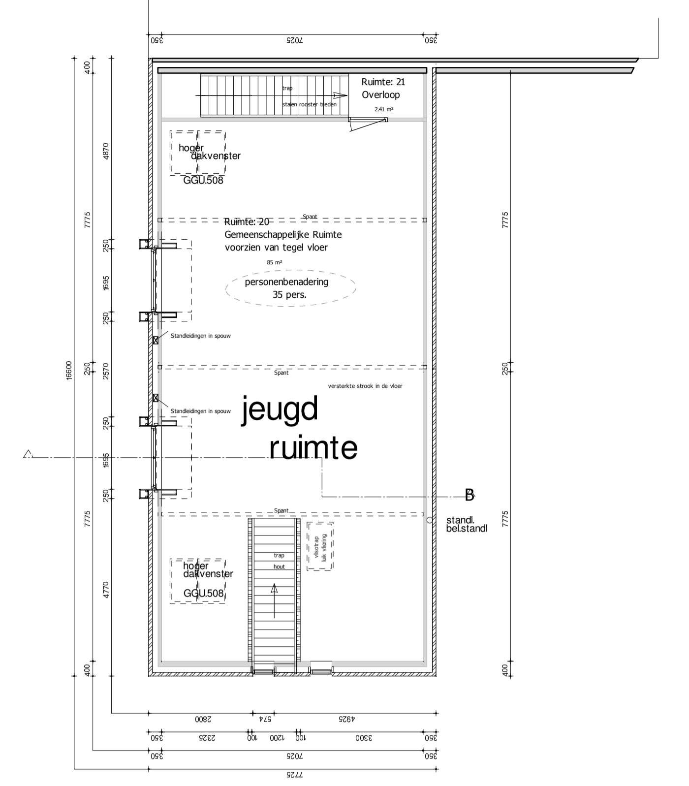
VERDIEPING
